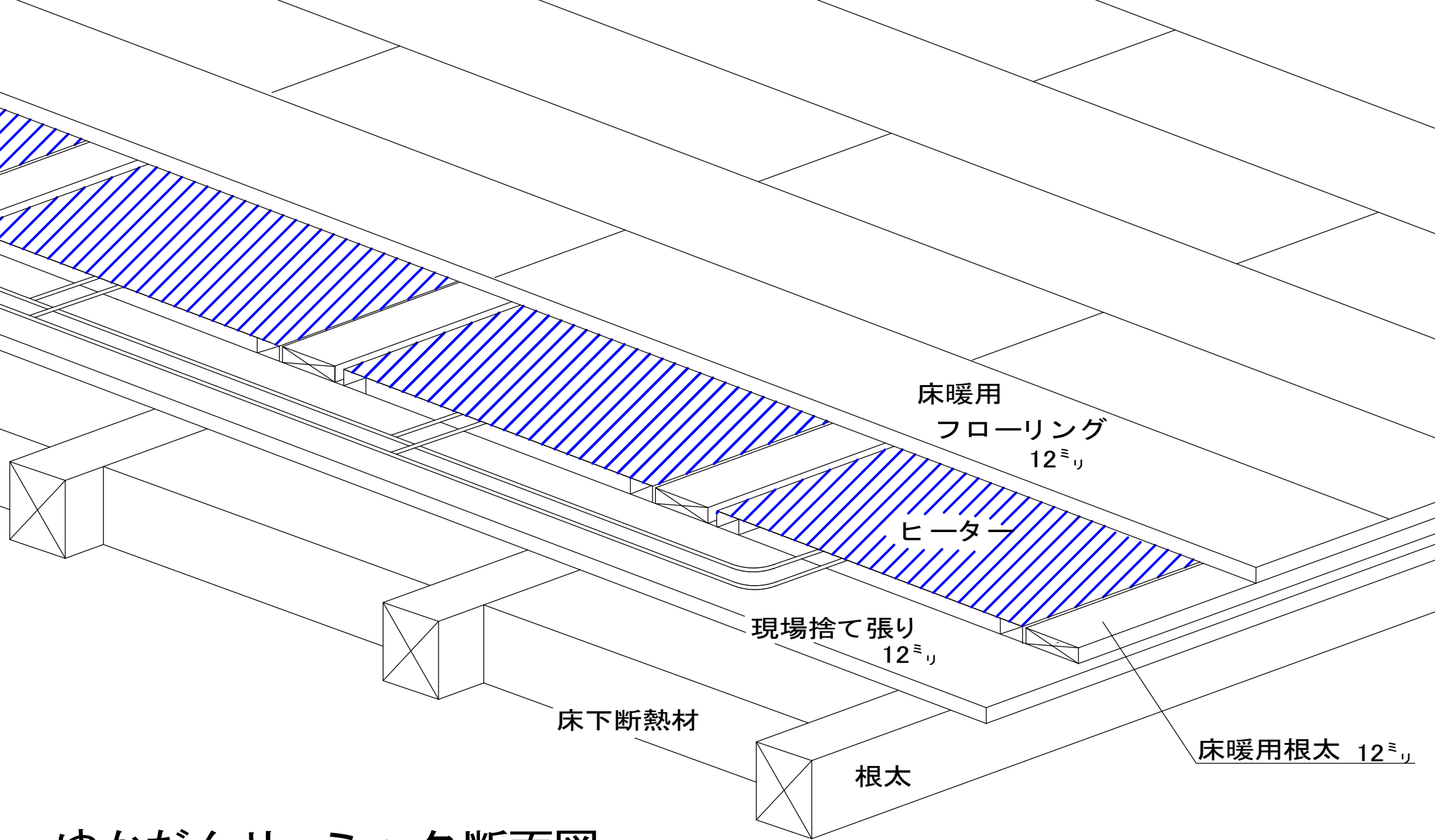
ゆかたんサーミック断面図
